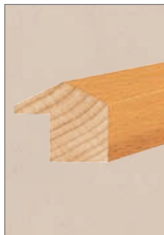
Glasleiste GDF Abmessung: 28 x 32 mm Falz: 17 x 12 mm Fixlängen: 2150 mm inkl. 2 Stoßlängen 1500 + 650 mm Menge pro Bund: 15 Stück
