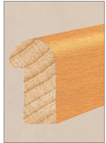
Soft-Line T S0 24 Abmessung: 20 x 36 mm Falz: 24 mm Fixlängen: 2150 mm inkl. 2 Stoßlängen Menge pro Bund: 15 Stück
