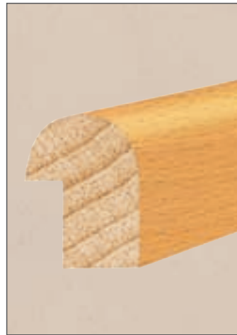
Soft-Line GT S0 Abmessung: 20 x 29 mm Falz: 17 mm Fixlängen: 2150 mm inkl. 2 Stoßlängen 1500 + 650 mm Menge pro Bund: 15 Stück
