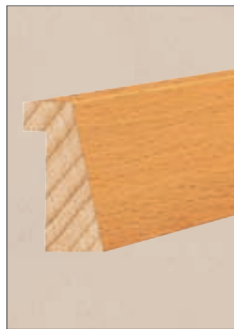
Bekleidungsleisten F 24 Falz 24 mm Fixlänge: 64,8 m = 24 Stück 2150 mm + 12 Stück 1100 mm oder 30 Stück 2150 mm nach unserer Wahl
