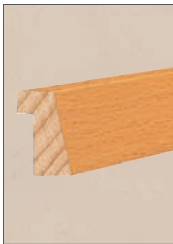
Bekleidungsleisten F 17 Falz 17 mm Fixlänge: 64,5 m inkl. Stoßlängen 1500 + 650 mm
