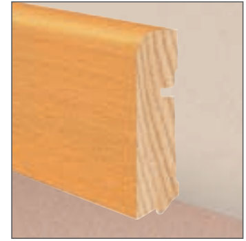
Sockelleiste 606 Deckfläche: 18 x 76/78* mm Fixlänge: 2700 mm / 2500 mm Menge pro Bund: 5 Stück Fallende Längen: 20 m
